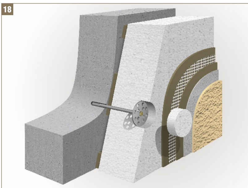
Rys. 18 - Montaż łączników mechanicznych w styropianie
