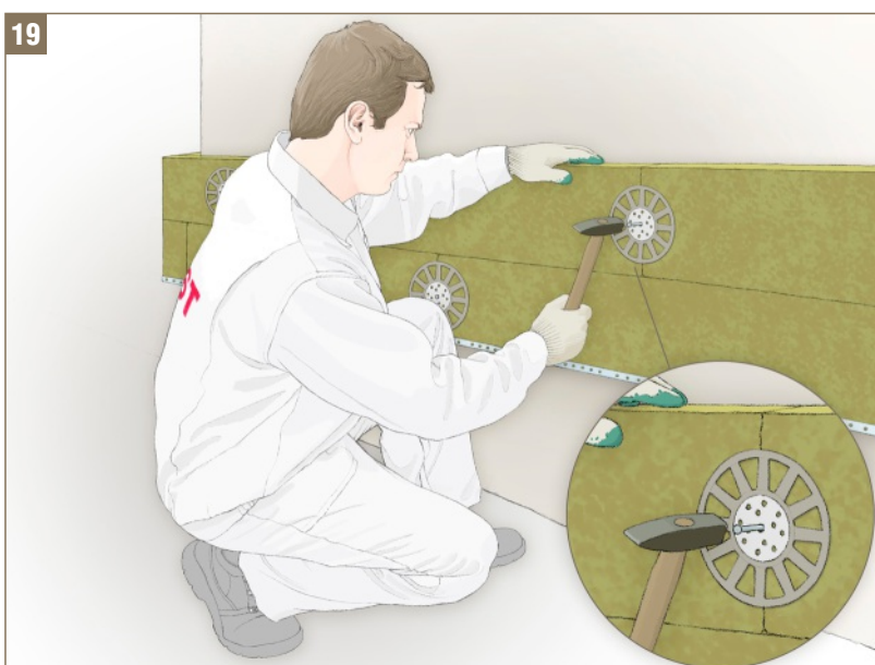
Rys. 19 - Montaż łączników mechanicznych na wełnie lamelowej
