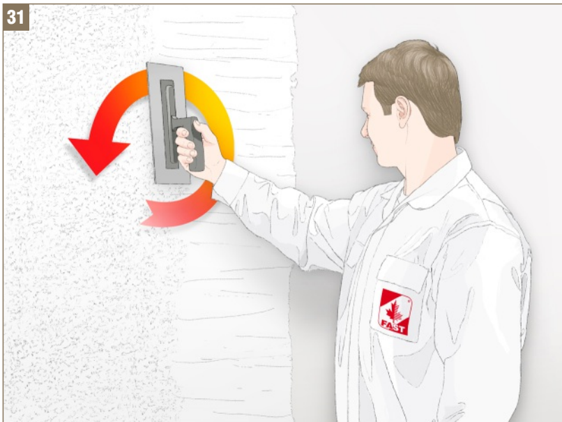
Rys. 31 - Zacieranie tynków - wykonywanie struktury baranka
