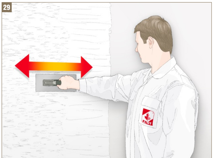
Rys. 29 - Zacieranie tynków - wykonywanie struktury kornika o rysach poziomych
