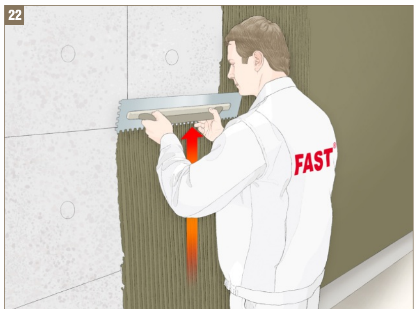
Rys. 22 - Nałożenie zaprawy klejowej packą grzebieniową
