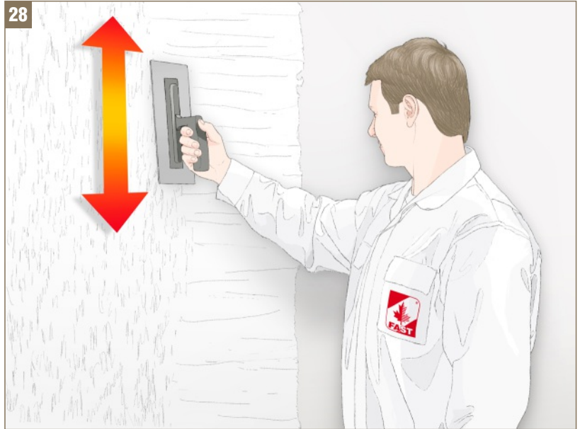
Rys. 28 - Zacieranie tynków - wykonywanie struktury kornika o rysach pionowych
